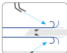
▲ 外捲模式 Up-roll : UC-L2/UC-L3 Mechanical & Automatic-Type
